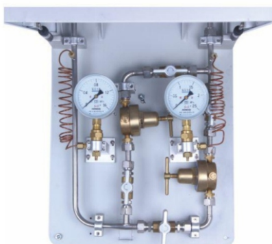
二级减压箱圆弧款
